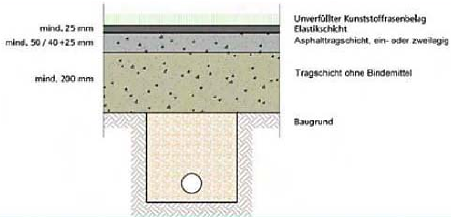
Abb. 114: Bauweise 3, Regelschnitt für unverfüllten Kunststoffrasenbelag mit Elastikschiicht auf Asphalttragschicht (Bauweise überwiegend bei Kombi-nutzung Hockey/Fußball)
