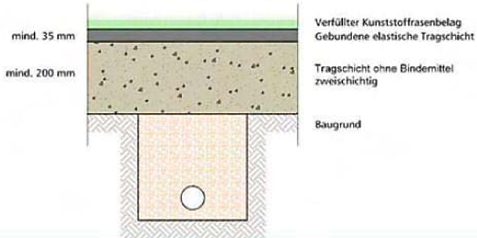
Abb. 112: Bauweise 1, Regelschnitt für gefüllten Kunststoffrasenbelag auf gebundener elastischer Tragschicht
