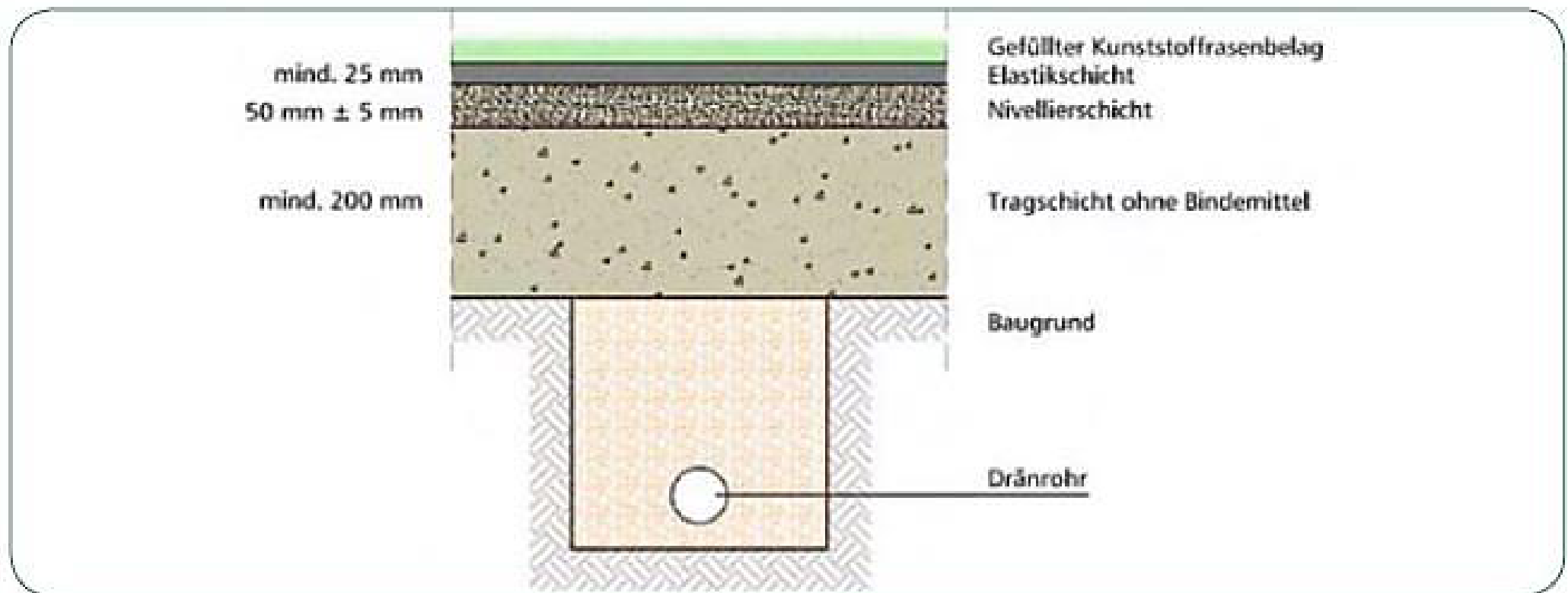
Abb. 113: Bauweise 2, Regelschnitt für gefüllten Kunststoffrasenbelag, Elastikschiicht auf Tragschiicht ohne Bindemittel und zusätzlicher Nivellierschiicht.
